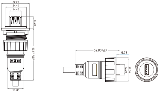
■ USB Cable connector
